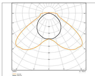
DP MAX DA 1200 S 43W 840 VW IP69
