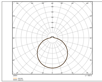
SF FLAT RD 330 P 19W ML 83040
