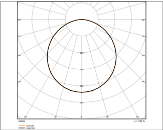
PL FLEX 625 S 32W 840 PS
